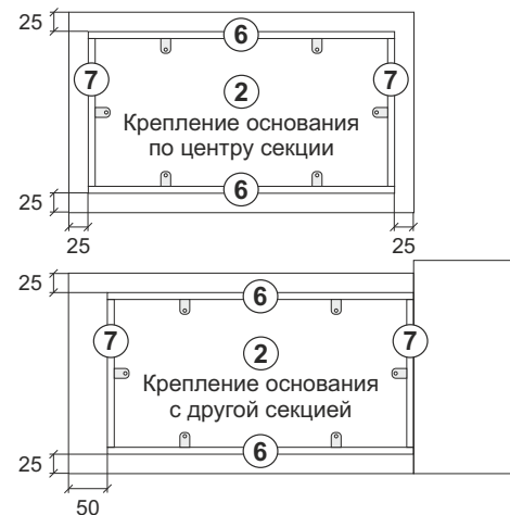
Рис.2 Вид снизу
