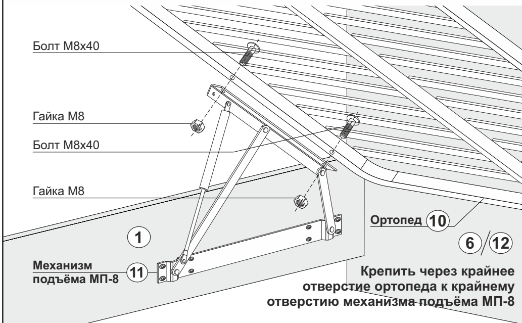
Рис.3: Монтаж механизма подъёма МП-8 (11) к ортопеду (10)
