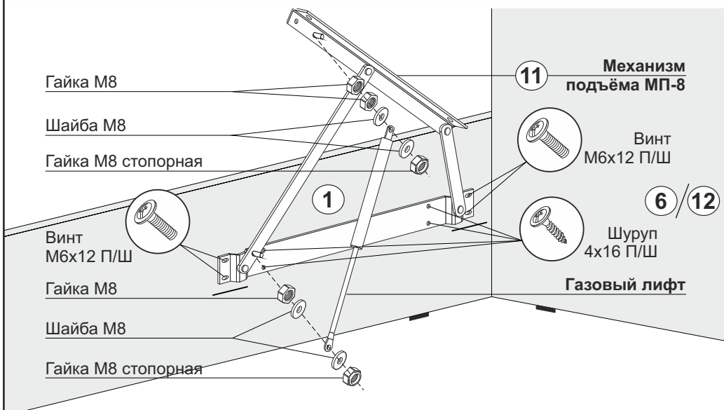
Рис.2: 1. Монтаж механизма подъёма МП-8 (11) к царгам (1) 2. Установка газового лифта на механизма подъёма МП-8 (11)
