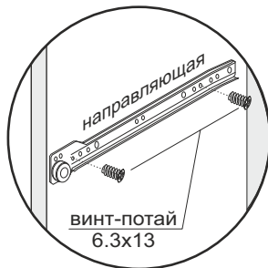
Рис.2 Сборка выдвижного ящика
