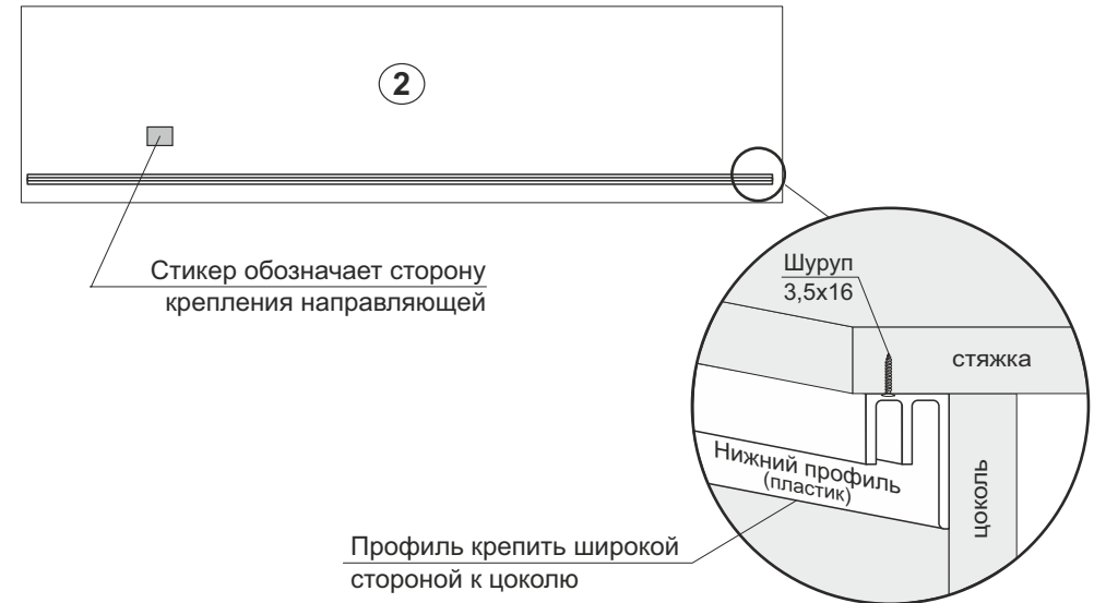
Рис.4 Монтаж нижней направляющей
