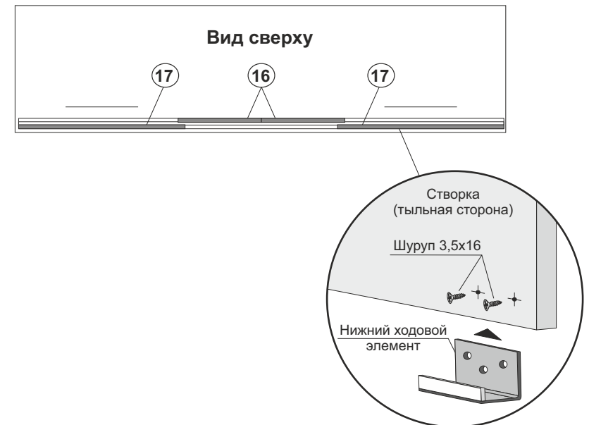
Рис.5 Монтаж нижнего ходового элемента
